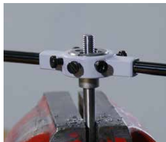
Außengewinde schneiden Cut external threads
