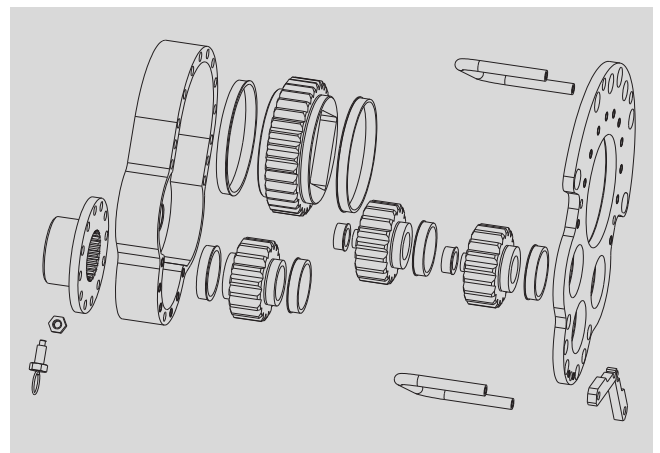
Zeichnung Getriebe drawing transmission
