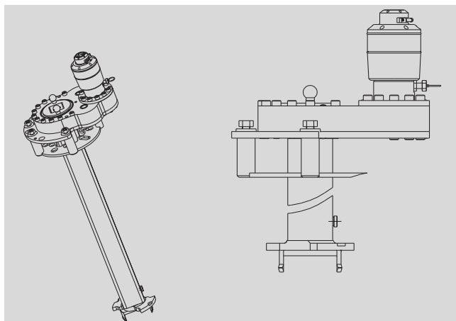
Seitenge triebe mit Boltmax Gerät Transmission with Boltmax Tool
